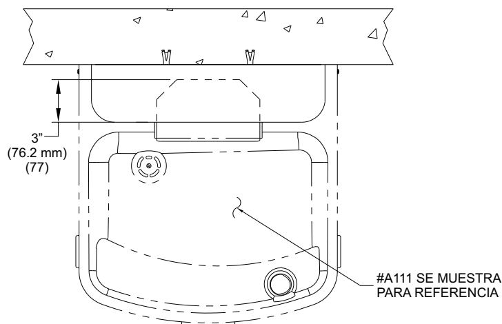
VISTA SUPERIOR
