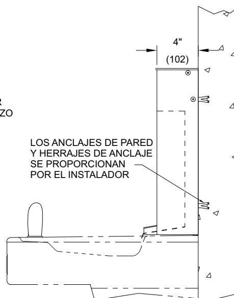
VISTA LATERAL
